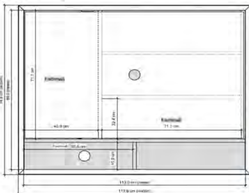
Panel schwenkbar links oder rechts
