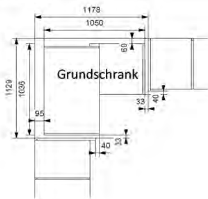
90° Ecke, 2-türig
